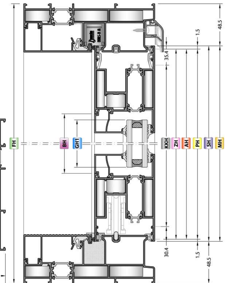
B-B SECTION / B-B KESİTİ
