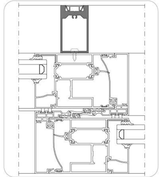
Application Details / Uygulama Detayı
