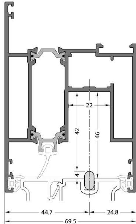
Univesal Lift & Slide Accesories Groove Universal Kaldır-Sür Aksesuar Kanalı
